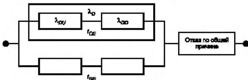
Рисунок В.6 — Схема расчета надежности архитектуры 1oo2
