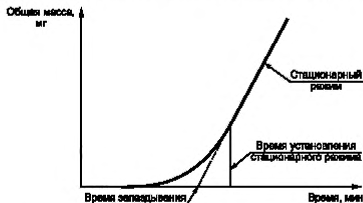
Рисунок 4 — Общий вид графика изменения общей массы продиффундировавшей испытательной жидкости во времени
