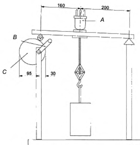
A – образец; B – кривошип; C – эксцентрик
