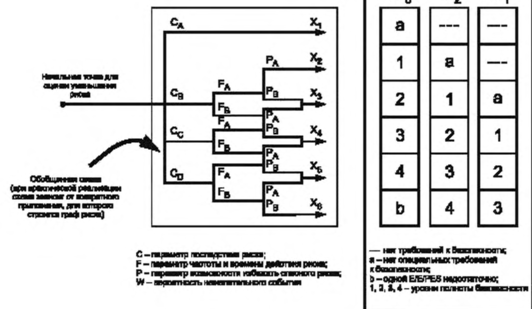
Рисунок D.1 — Граф риска: общая схема
