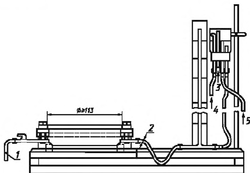
1 — выпуск воздуха; 2 — трубка внутренним диаметром не менее 6 мм; 3 — выпуск воздуха; 4 — выпуск воды; 5 — выпуск воды
