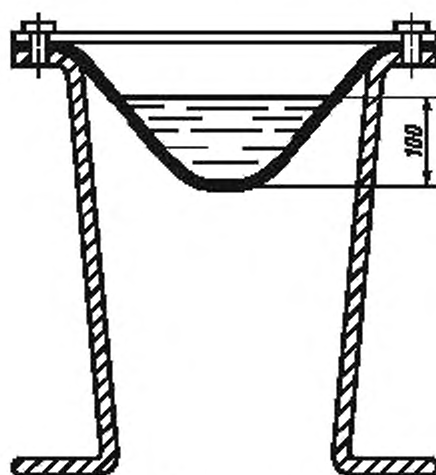
Рисунок 4 — Приспособление для определения водопроницаемости методом кошеля
