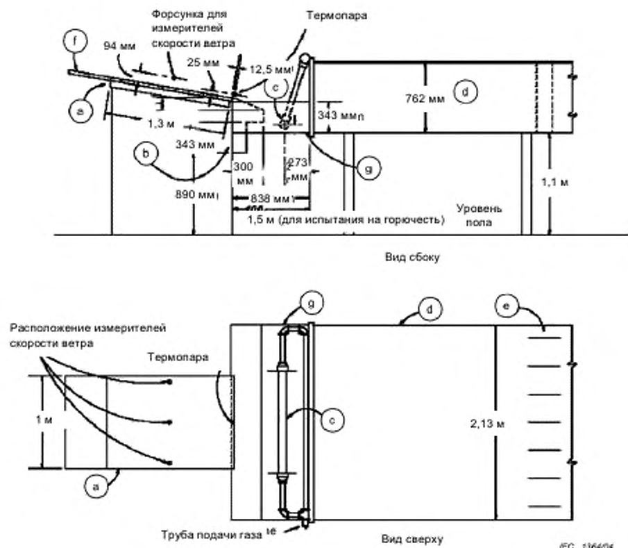
Рисунок А.1 — Конструкция для испытания на огнестойкость
