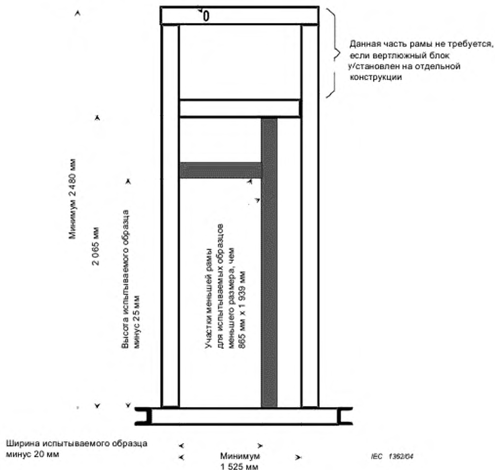
Рисунок 6 — Конструкция № 2 для испытания на удар
