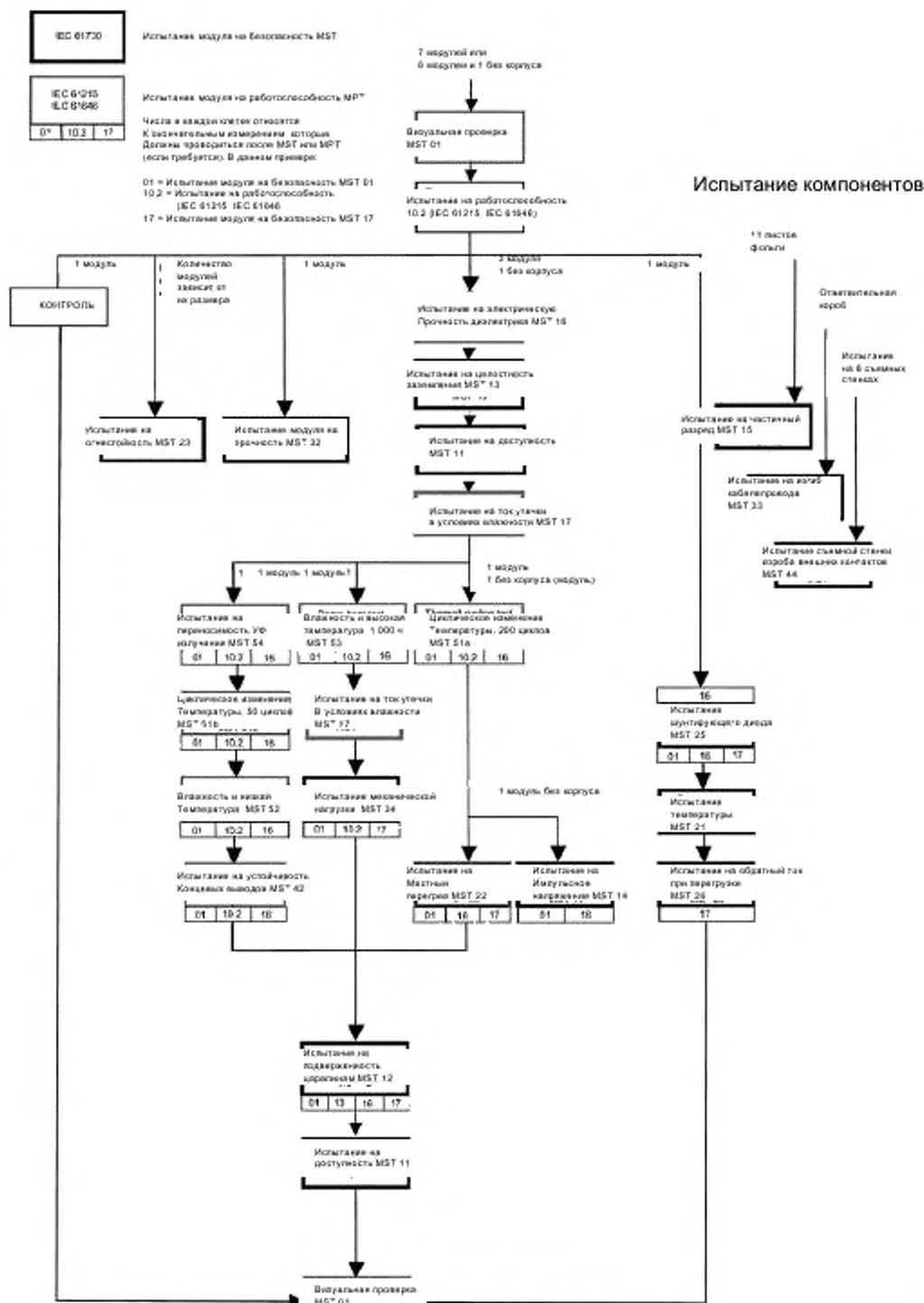
Рисунок 1 — Схема испытаний
