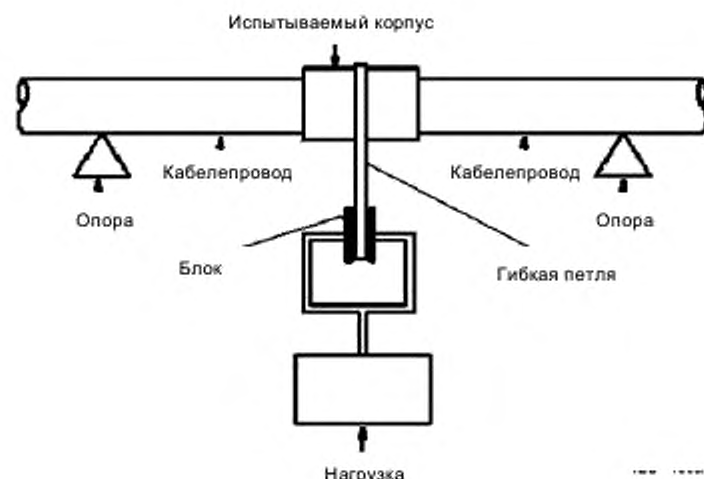
Рисунок 7 — Испытательное приспособление в сборе
