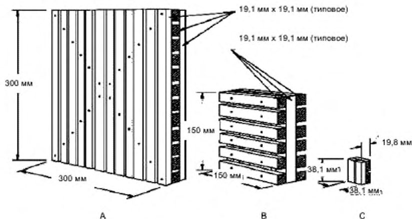
Рисунок А.2 — Конструкция для испытания на горючесть
