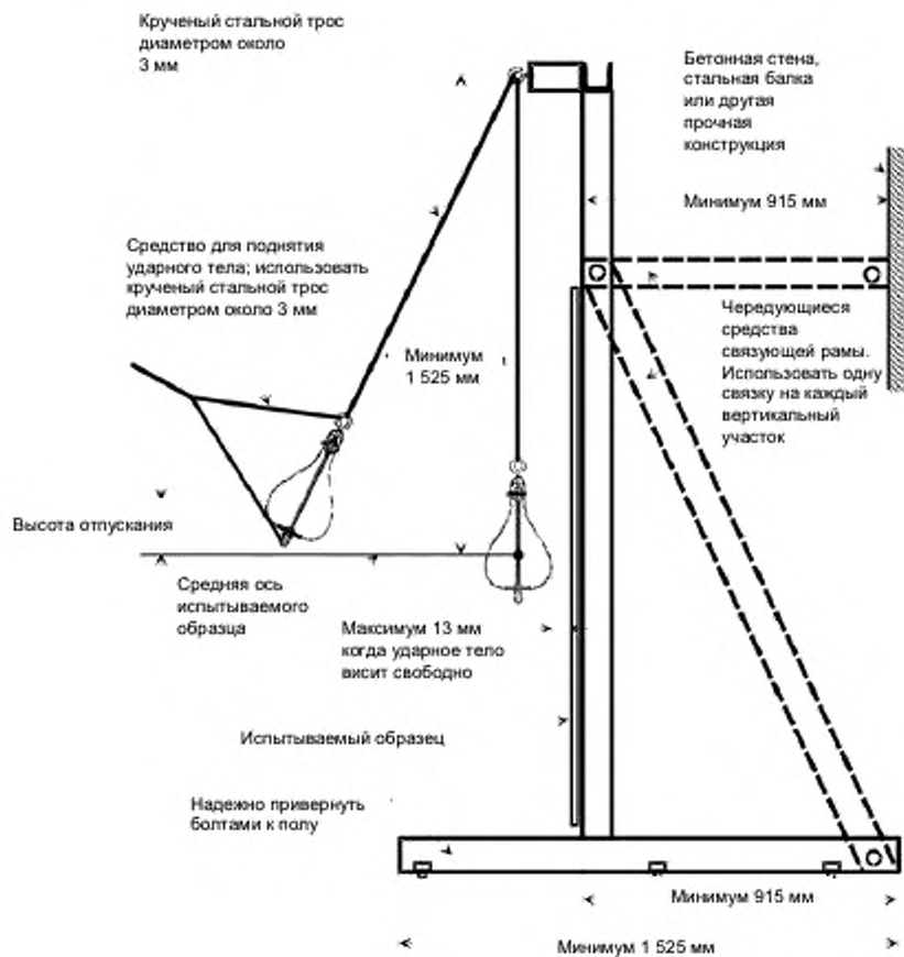
Рисунок 5 — Конструкция № 1 для испытания на удар
