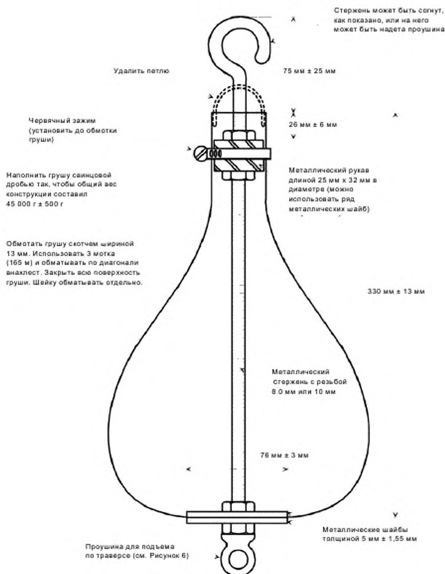
Рисунок 4 — Ударная груша
