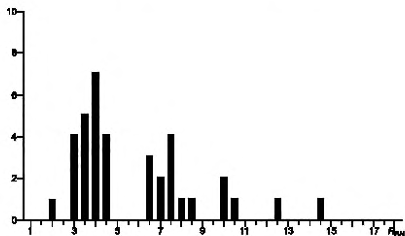
Рисунок А.2 Гистограмма распределений значений R_{BN} для 37 лечебных головок различных диаметров и частоты
