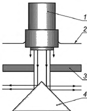
1 — лечебная головка; 2 — поверхность воды; 3 — апертурная маска; 4 — мишень измерителя радиационной силы
