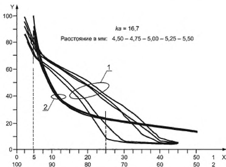
Рисунок D.1 — Линии равных давлений типовой физиотерапевтической лечебной головки малой геометрической площади ( \lambda = 17 )
