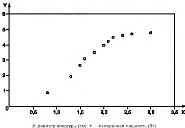
Рисунок I.2 — Измеренная мощность, прошедшая через апертуры различного диаметра, для лечебной головки с частотой 1 МГц
