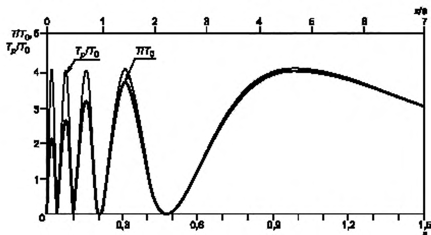
Рисунок А.1 Осевая зависимость нормированной усредненной по времени акустической интенсивности (сплошная линия) и ее плоско-волновой аппроксимации (штриховая линия) для круглого поршневого излучателя с ka = 30 от нормированного расстояния s (где s = \lambda z/a^2 )
