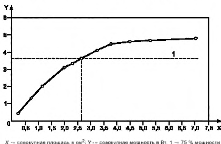
Рисунок 1.3 — Совокупная сумма кольцевых вкладов мощности, предварительно отсортированных в порядке убывания вкладов интенсивности, в зависимости от совокупной суммы площадей соответствующих колец
