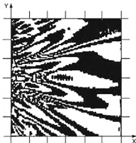
Рисунок D.1 — Линии равных давлений типовой физиотерапевтической лечебной головки малой геометрической площади ( \lambda = 17 )
