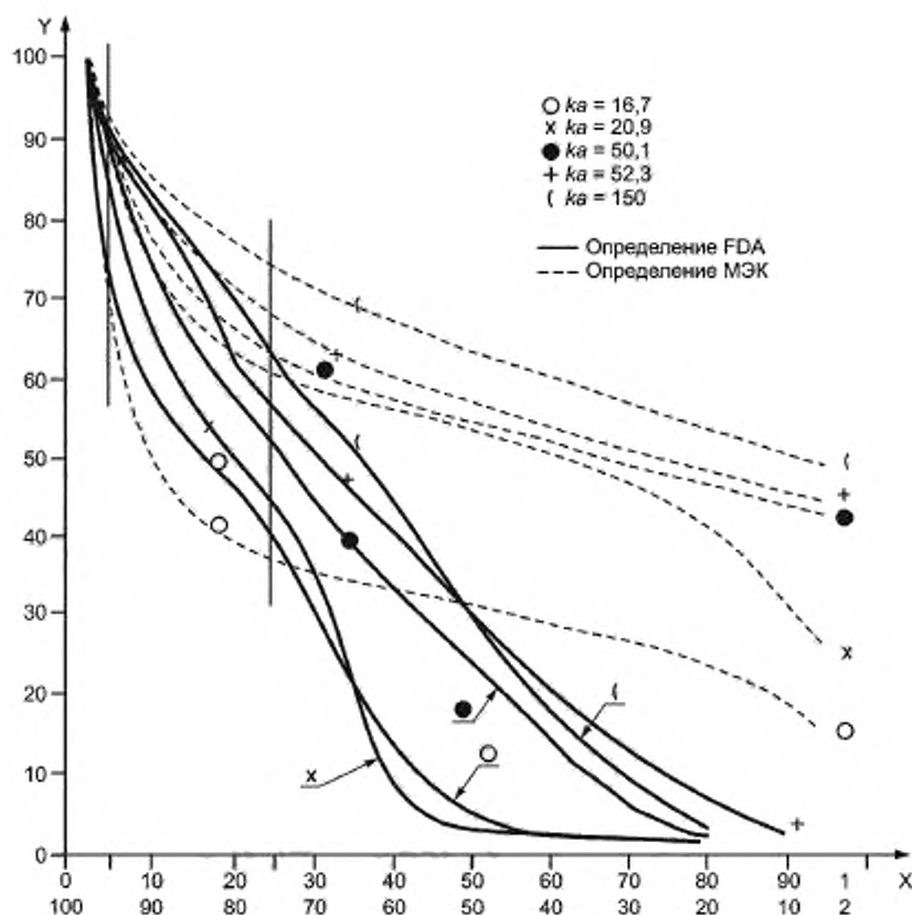
Рисунок D.3 — Нормированные значения площади поперечного сечения пучка при ограничениях FDA и МЭК для 5 преобразователей с различными ka при z = 0,5 см
