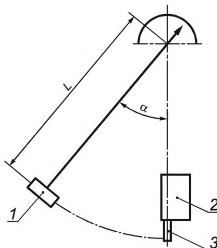
1 — масса; 2 — ПК в присоединенном положении; 3 — испытательные торцевые соединения в закрытом положении
