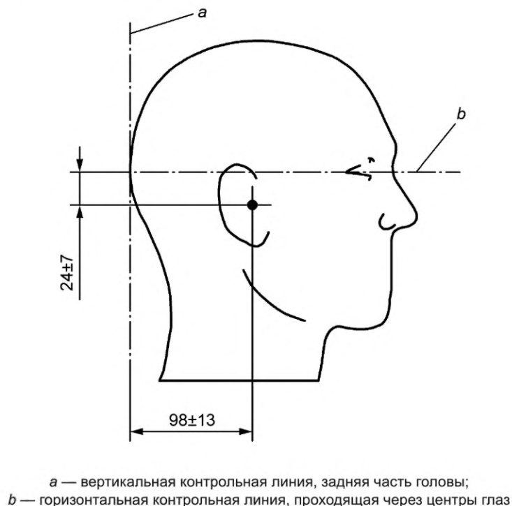
Рисунок 11 — Расположение микрофонов
