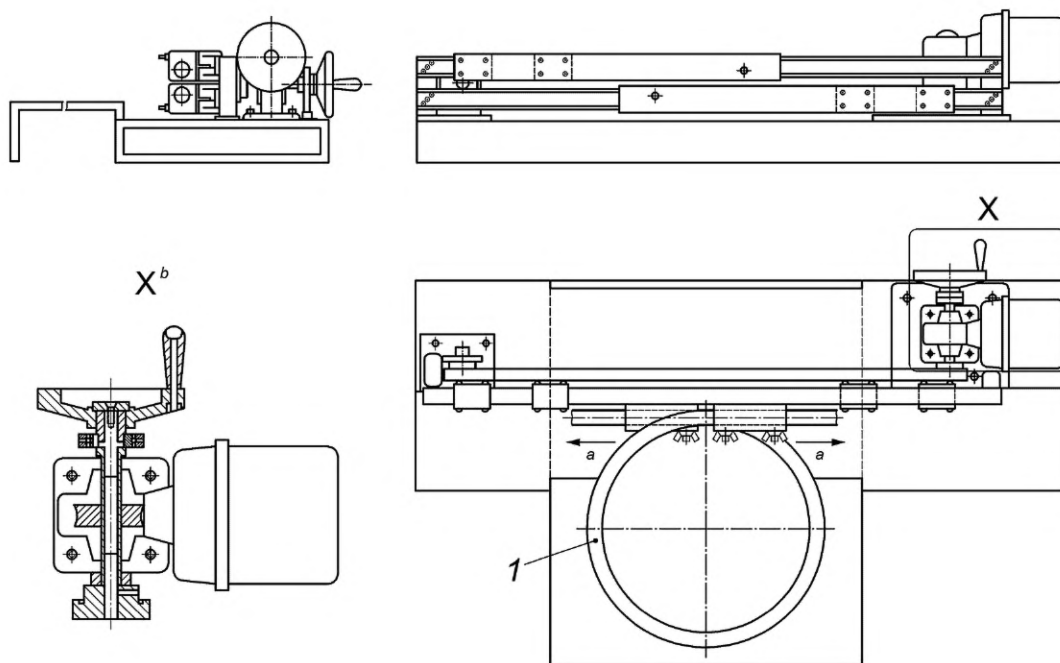
1 — шланг; а — направление движения; b — сечение детали X
