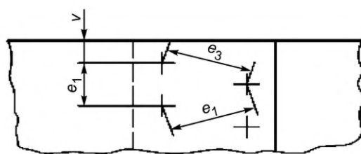
Рисунок F.3 — Контактная точечная сварка листового металла, двухрядная
