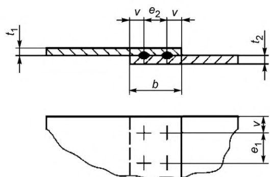
Рисунок F.2 — Контактная точечная сварка листового металла, однорядная
