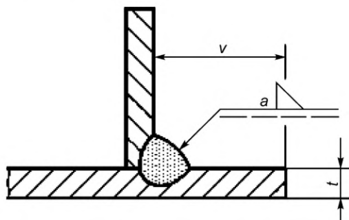
Рисунок 11 — Расстояние от края для угловых швов
