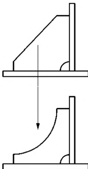
Рисунок 9 — Форма косынок
