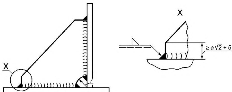
Рисунок 8 — Проектирование концов косынок и фасонных элементов жесткости
