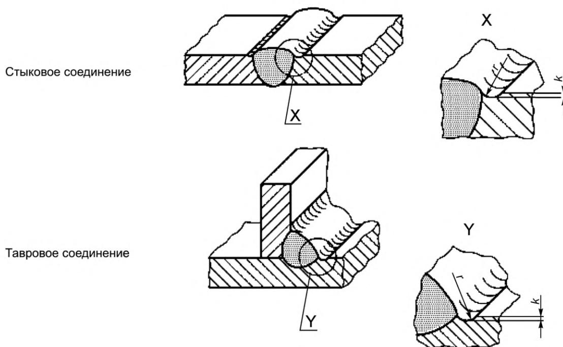
Рисунок 17 — Улучшение границы сварного шва
