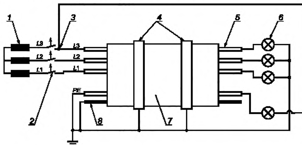
1 — трансформатор; 2 — плавкий предохранитель (2 А); 3 — подсоединение к линии L3 (или L1 , или L2 ); 4 — поддерживающие кольца; 5 — испытуемая жила или группа жил; 6 — нагрузочный индикаторный прибор (например, лампа); 7 — образец; 8 — металлический экран (если имеется); L1 , L2 , L3 — линии испытуемых жил или групп жил ( L2 , L3 , если имеются); PE — жила заземления (если имеется)
