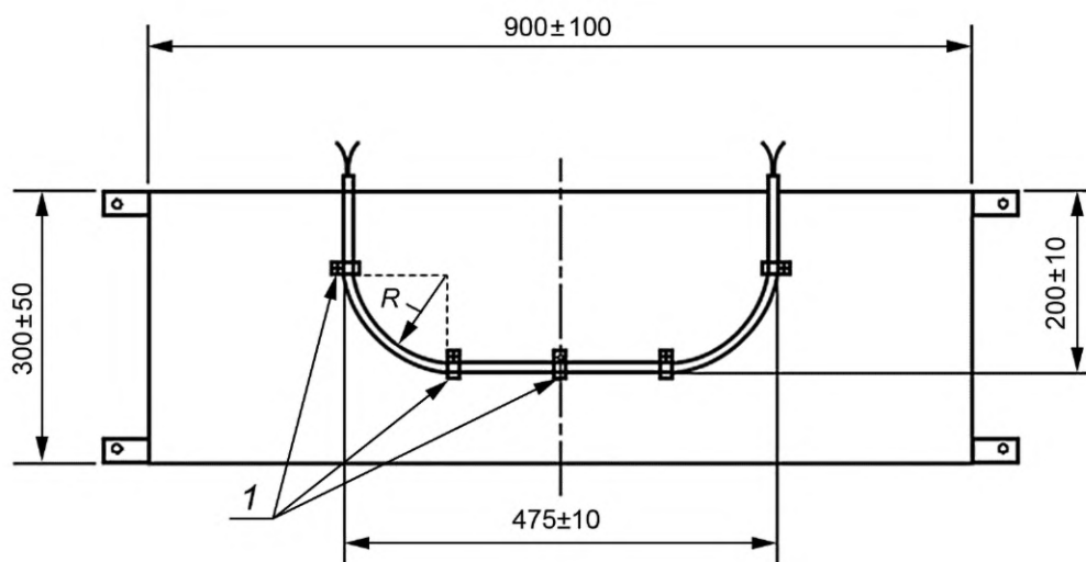
Рисунок 7 — Способ крепления образца при испытании
