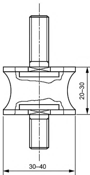
Рисунок 4 — Типичная резиновая втулка для крепления испытательной стенки
