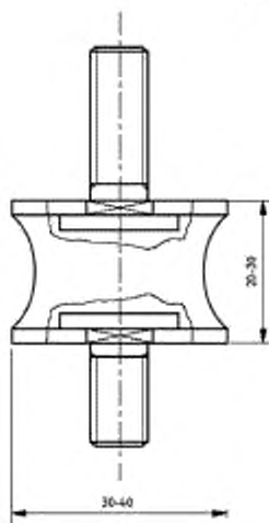
Рисунок 5 — Типичная резиновая втулка для крепления испытательной лестницы
