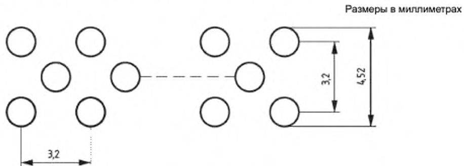
Рисунок 6 — Фронтальная поверхность рабочей части горелки
