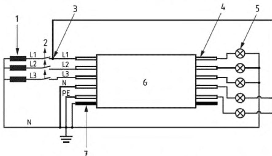
1 — трансформатор; 2 — плавкий предохранитель (2 А); 3 — фазы L1, L2 или L3; 4 — испытуемая жила или группа жил; 5 — нагрузочный индикаторный прибор; 6 — образец; 7 — металлический экран (при наличии); L1, L2, L3 — фазные жилы (L2, L3 при наличии); N — нейтральная жила (при наличии); PE — защитная жила (при наличии)
