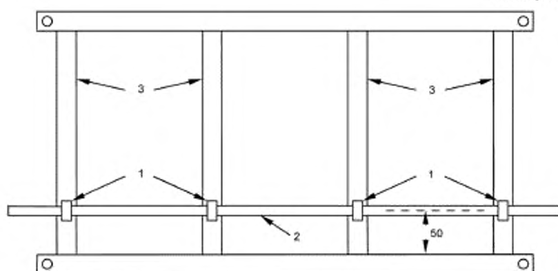
Рисунок 2 — Рекомендуемый способ крепления металлического корпуса испытательной лестницы
