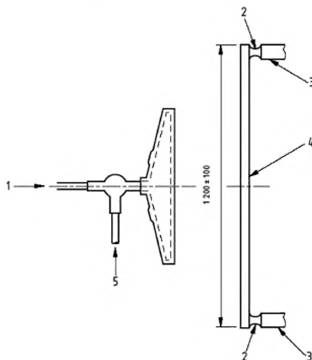
Рисунок 2 — Рекомендуемый способ крепления металлического корпуса испытательной лестницы
