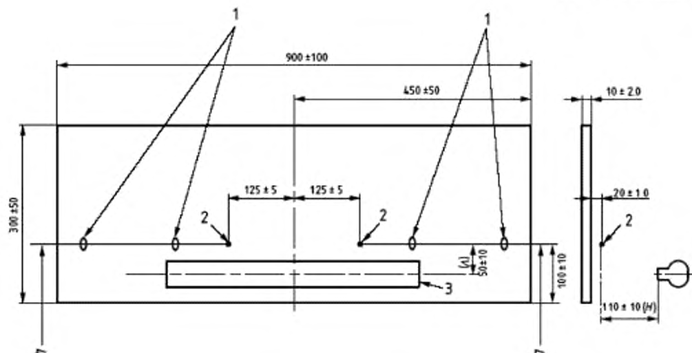
1 — опоры для термопар; 2 — кончик термопары; 3 — горелка; 4 — термопара типа К; H — расстояние кончика термопары от фронтальной поверхности горелки по горизонтали; V — расстояние до кончика термопары от осевой линии горелки по вертикали
