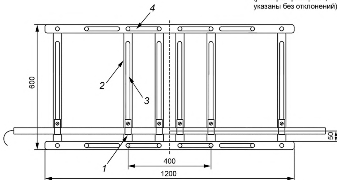
1 — P-образный хомут; 2 — регулируемые вертикальные элементы; 3 — прорезь для крепления P-образного хомута; 4 — прорезь для перемещения регулируемых вертикальных элементов
