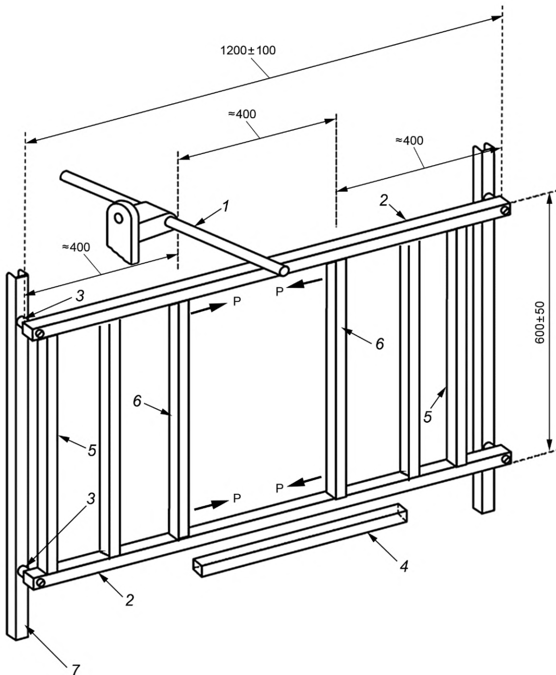
1 — ударное устройство; 2 — стальная испытательная лестница; 3 — резиновая втулка; 4 — газовая горелка ленточного типа; 5 — неподвижный вертикальный элемент; 6 — регулируемый вертикальный элемент; 7 — жесткий опорный каркас; P — плоскость регулировки
