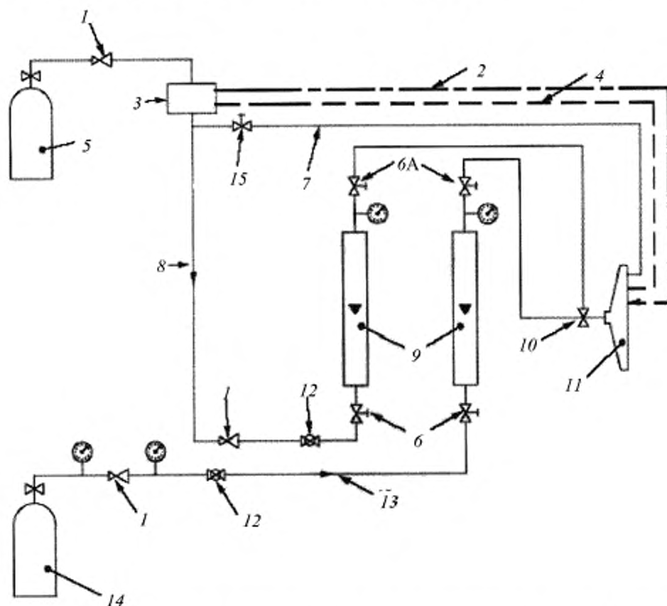
1 — редуктор; 2 — пьезоэлектрический воспламенитель; 3 — устройство для прерывания работы горелки; 4 — контрольные термодатчики; 5 — баллон с пропаном; 6 — винтовой клапан (6А — альтернативное расположение); 7 — вспомогательное питание; 8 — поступление газа; 9 — расходомер типа ротаметр; 10 — смеситель Вентури; 11 — горелка; 12 — шаровый вентиль; 13 — поступление воздуха; 14 — баллон со сжатым воздухом; 15 — винтовой клапан предпускового питания
