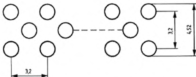
Рисунок 5 — Фронтальная поверхность рабочей части горелки
