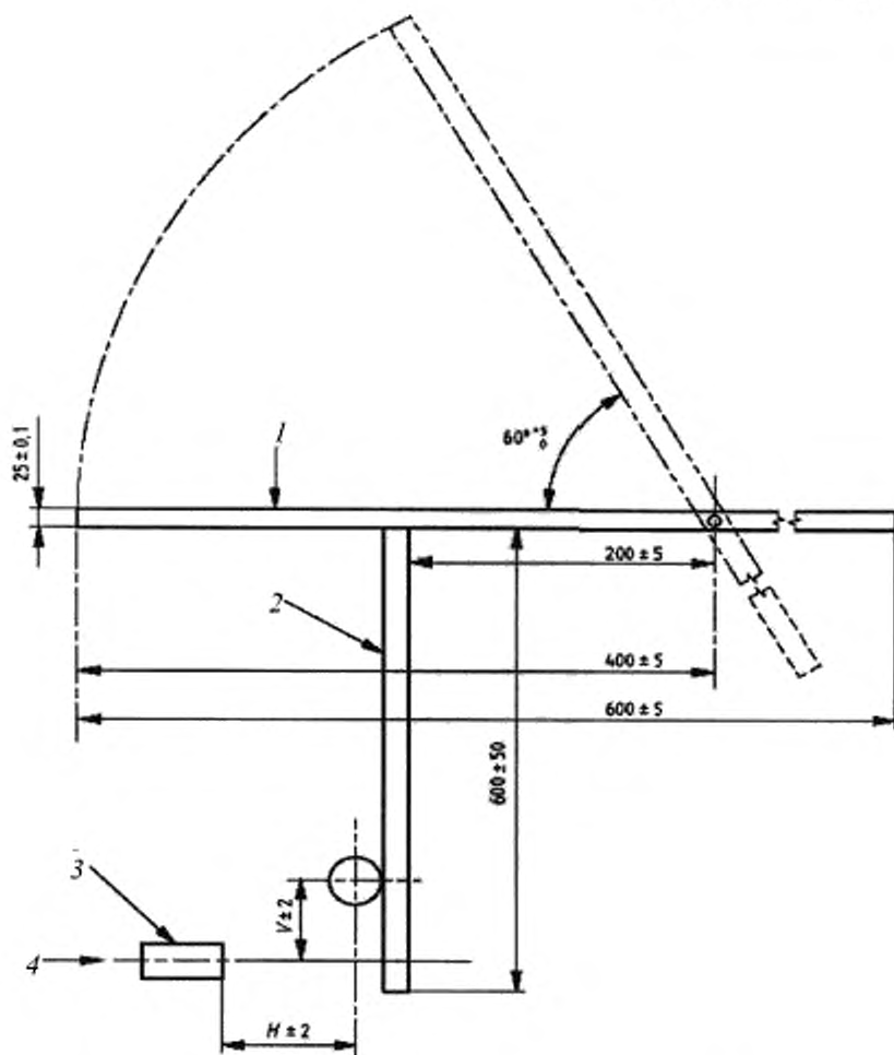
1 — ударное устройство; 2 — стальная испытательная лестница; 3 — газовая горелка; 4 — осевая линия фронтальной поверхности горелки; H — расстояние по горизонтали от осевой линии испытуемого кабеля до фронтальной поверхности горелки; V — расстояние по вертикали от осевой линии испытуемого кабеля до осевой линии горелки
