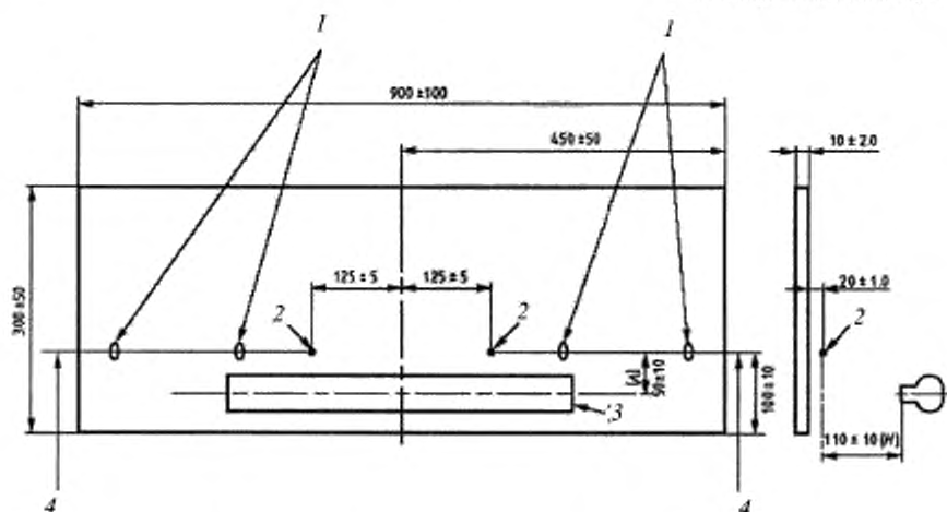
1 — опоры для термопар; 2 — кончик термопары; 3 — горелка; 4 — термопары типа К; Н — расстояние до кончика термопары от фронтальной поверхности горелки по горизонтали; V — расстояние до кончика термопары от осевой линии горелки по вертикали
