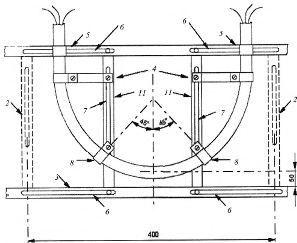
1 — отрегулированное положение вертикальных элементов; 2 — исходное положение вертикального элемента; 3 — нижний горизонтальный элемент испытательной лестницы; 4 — дополнительный зажим для обеспечения дугообразной формы кабеля (при необходимости); 5 — U-образный хомут; 6 — прорезь для перемещения регулируемых вертикальных элементов; 7 — прорезь для крепления P-образного хомута; 8 — P-образный хомут
