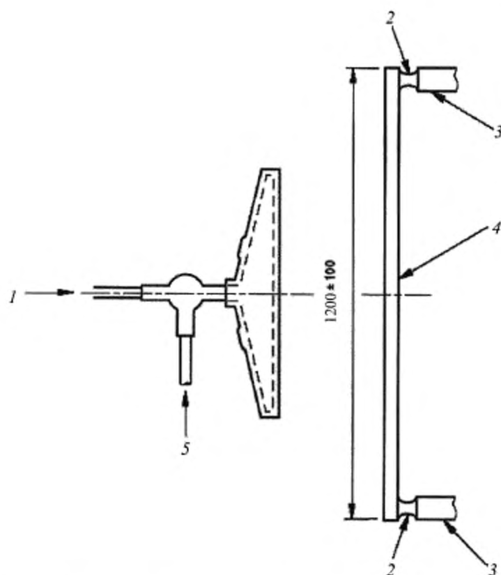
Рисунок 2 — Испытательное устройство (вид сверху)
