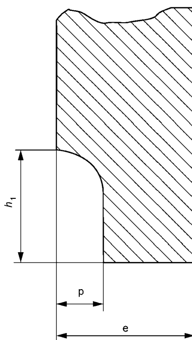
Рисунок 6 — Скол — вид с торца
