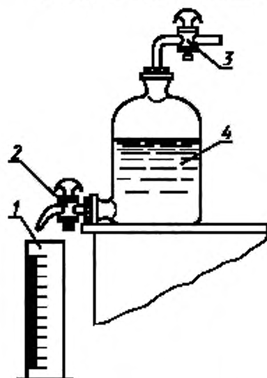
Аспиратор с измерительным цилиндром
