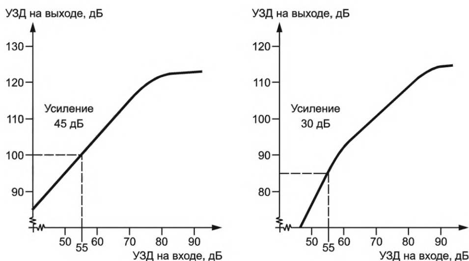
Рисунок 2 — Примеры кривых отклика «вход-выход» при частоте 1 кГц и определение усиления при входном УЗД 55 дБ
