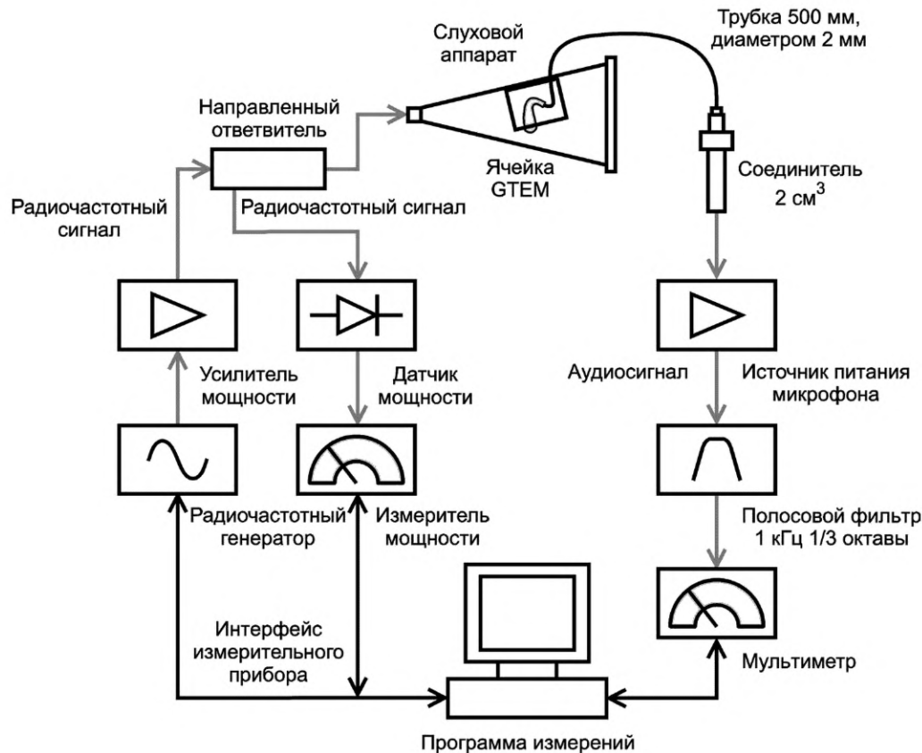
Рисунок 1 — Пример испытательной установки для измерения устойчивости слухового аппарата с использованием ячейки GTEM
