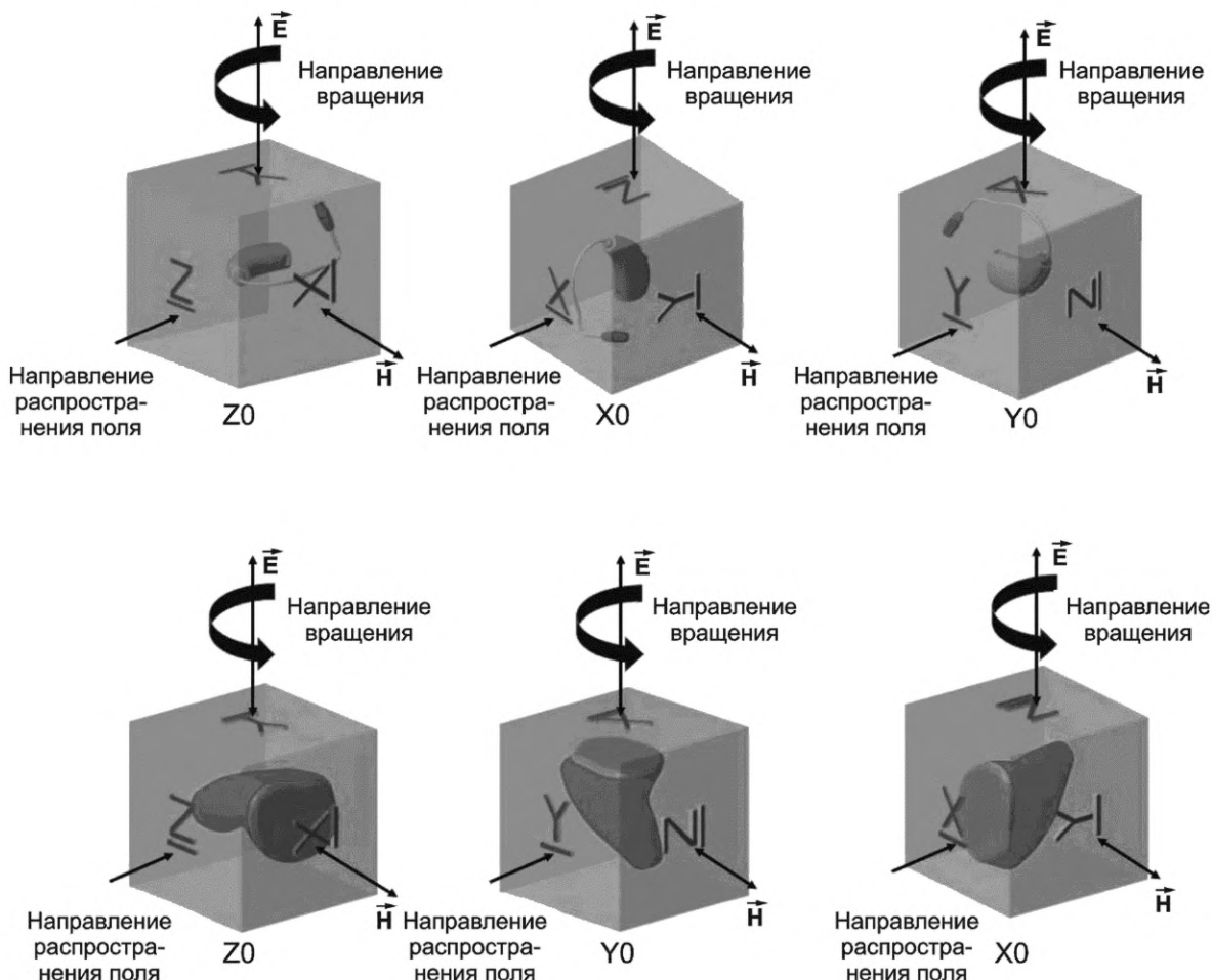
Рисунок 3 — Испытательные положения слухового аппарата для ВТЕ (вверху) и ИТЕ (внизу)
