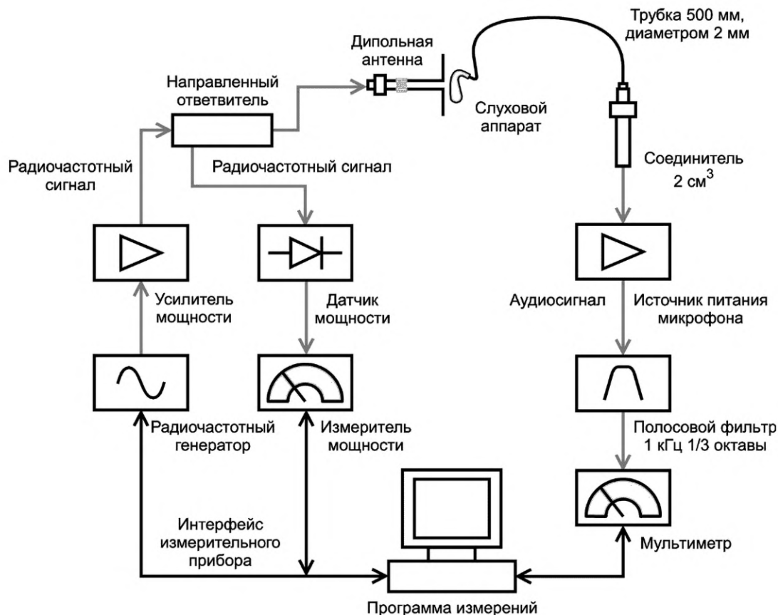
Рисунок А.2 — Пример испытательной установки для измерения устойчивости к помехам слухового аппарата с использованием дипольной антенны
