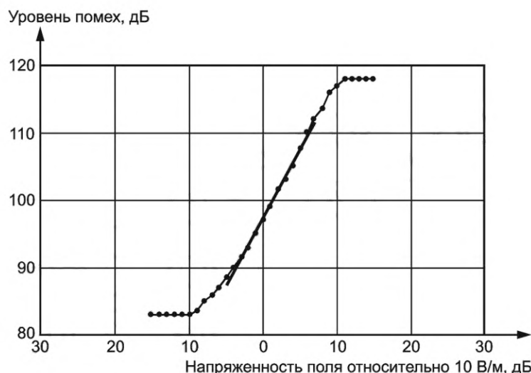
Рисунок А.1 — Соотношение 1:2 между напряженностью поля и уровнем помех в децибелах
