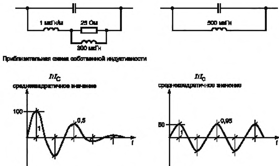
Рисунок 5 — Оборудование для демпфирования и ограничения тока с демпфирующим резистором и без него
