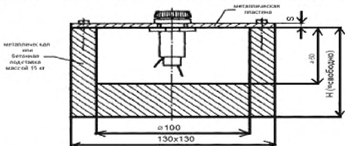
Размеры в миллиметрах Рисунок 6 — Испытательное устройство для технического испытания
