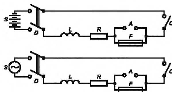
а) Испытательная схема для проверки отключающей способности плавких вставок с высокой и средней отключающей способностью
