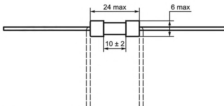
Рисунок А.2 — Испытательное основание
