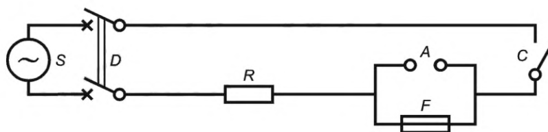
Рисунок 6 — Типовая испытательная схема для проверки отключающей способности плавких вставок с высокой отключающей способностью
