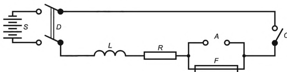
а) Типовая испытательная схема для испытаний отключающей способности плавких вставок с отключающей способностью выше 100 А
