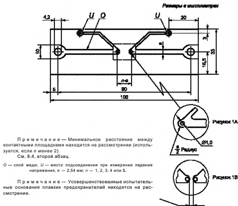
Рисунок 1 — Стандартная испытательная печатная плата (для номинальных токов до 5 А) (см. 7.3)
