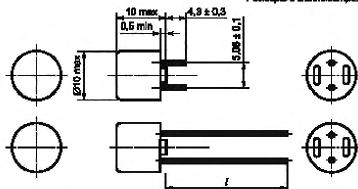
Размеры в миллиметрах
