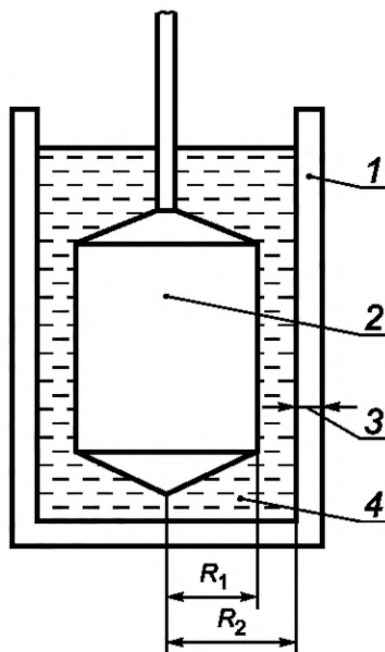
1 — контейнер для образца; 2 — шпindel; 3 — толщина испытуемого образца; 4 — испытуемый образец; R_1 — радиус шпинделя; R_2 — внутренний радиус контейнера для образца
