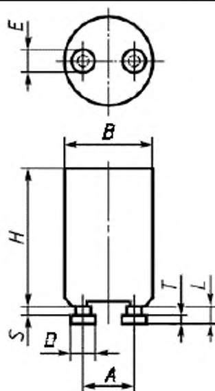
Рисунок 1 — Размеры стартеров
