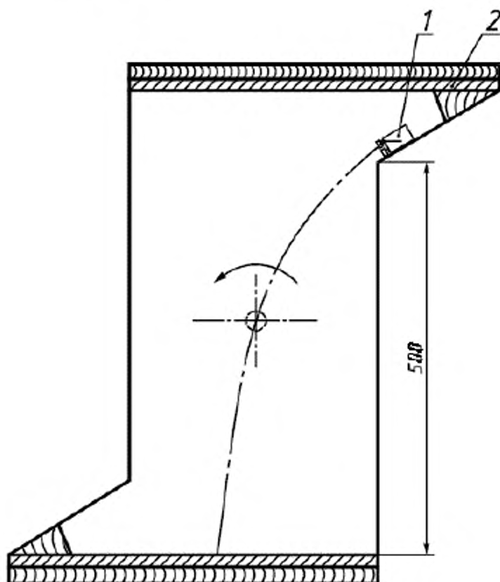
1 – стартер; 2 – стальная пластина
