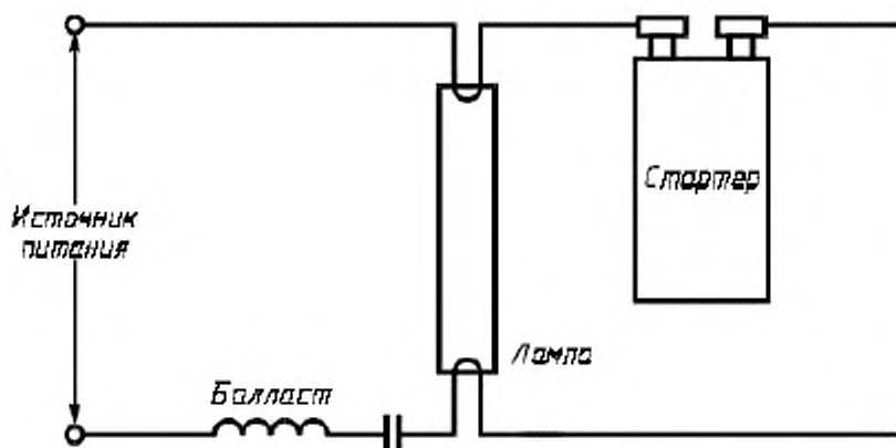
Рисунок 10 — Схема испытания стартеров на долговечность
