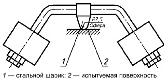
Рисунок 6 — Устройство для испытания вдавливанием шарика
