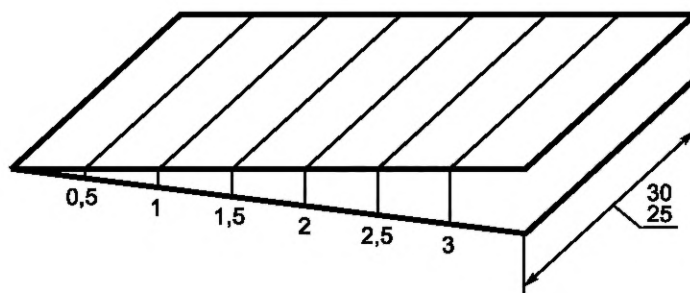
Рисунок 5 — Толщиномер клиновидной формы
