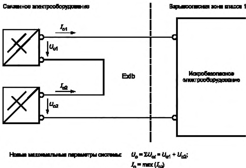
Рисунок I.1 — Последовательное соединение.
