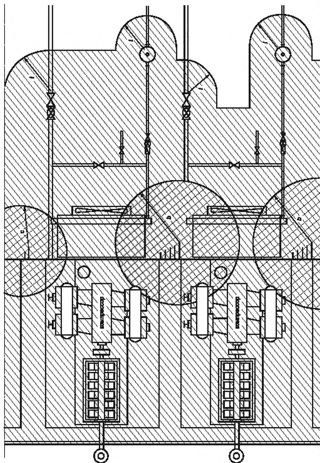
Рисунок D. 1a — Пример классификации зон для компрессора, работающего на природном газе
