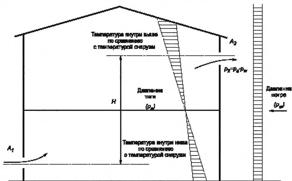
Рисунок C.1 — Пример противодействующих движущих сил вентиляционных потоков
