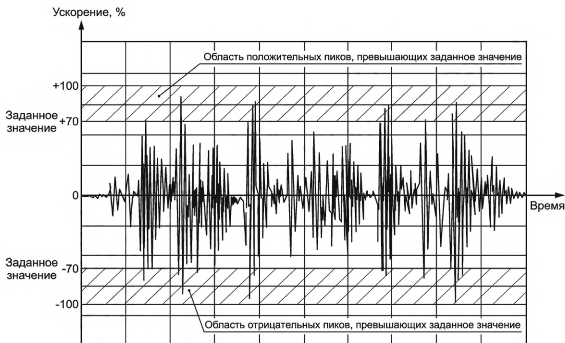
Рисунок 5 — Типичный отклик осциллятора на воспроизведенную акселерограмму процесса
