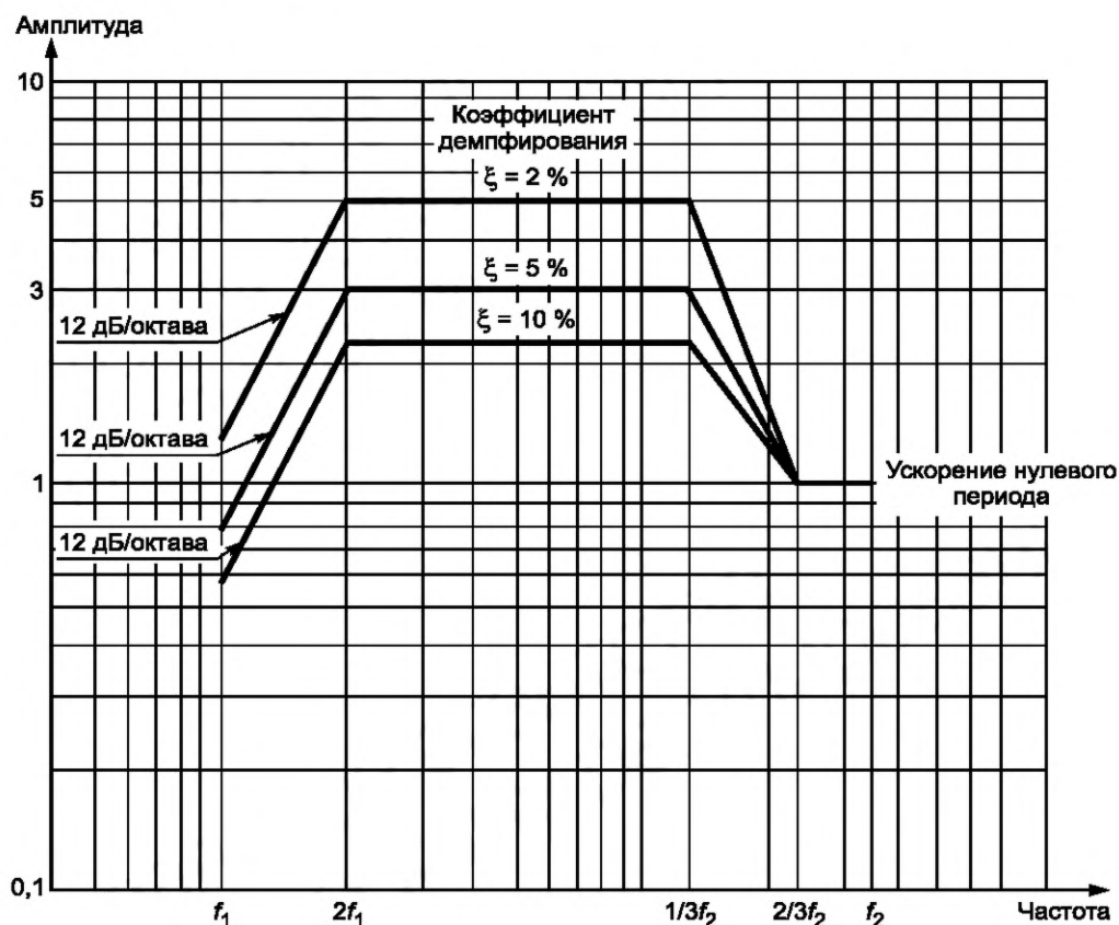
Рисунок А.1 — Рекомендуемая общая форма для заданного спектра отклика
