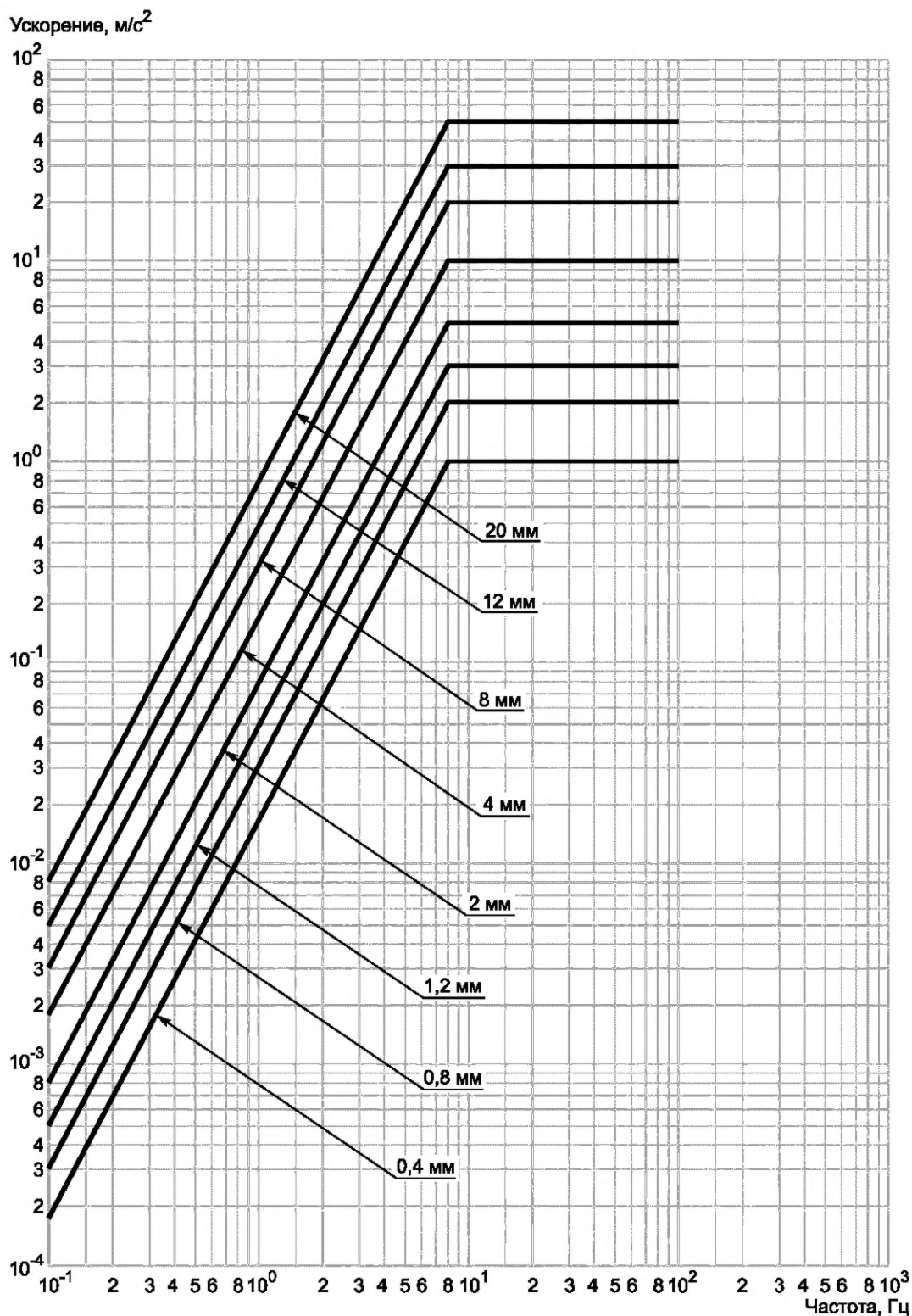
Рисунок 8 — Рекомендуемые уровни вибрации при частоте перехода 8 ц
