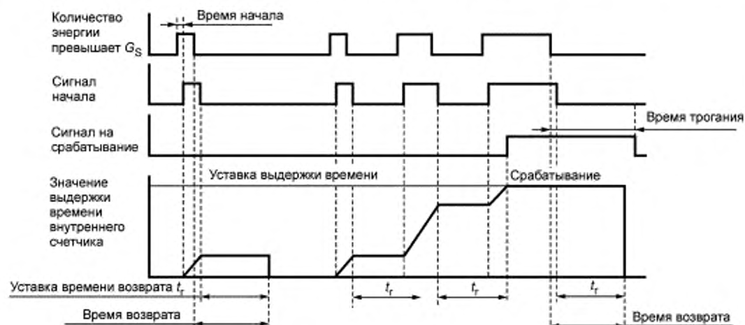
Рисунок 5 — Характеристика, поясняющая время возврата реле
