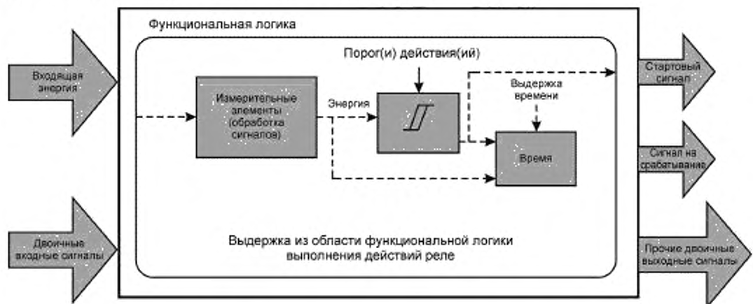
Рисунок 1 — Функциональный блок диаграмм выполнения защиты
