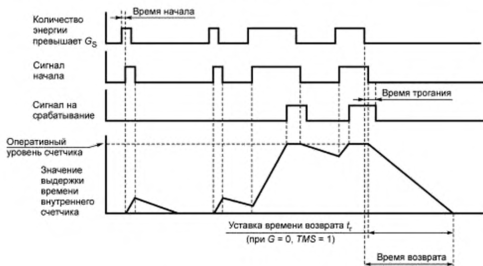
Рисунок 7 — Зависимая характеристика времени возврата
