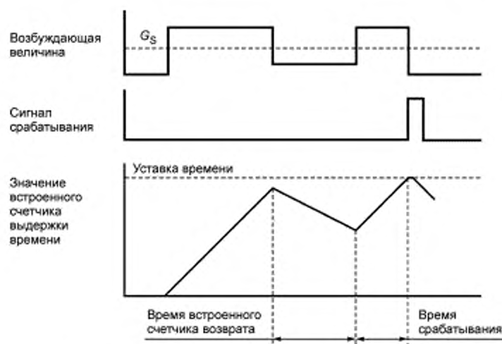
Рисунок В.1 — Определение зависимости времени возврата
