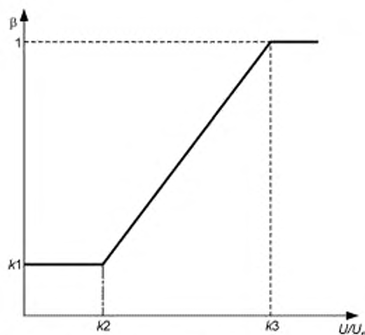
Рисунок 9 — Характеристика ограничения напряжения
