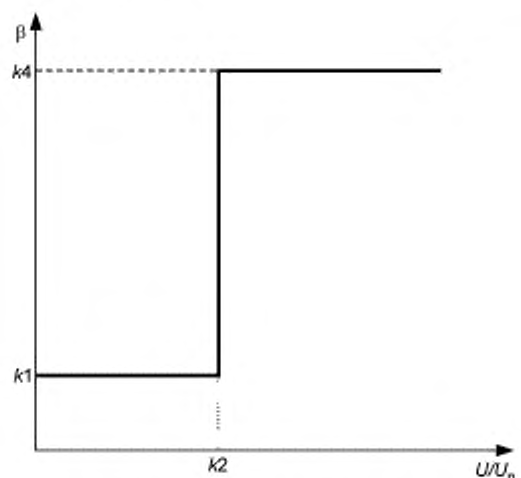
Рисунок 10 — Характеристика управляющего напряжения
