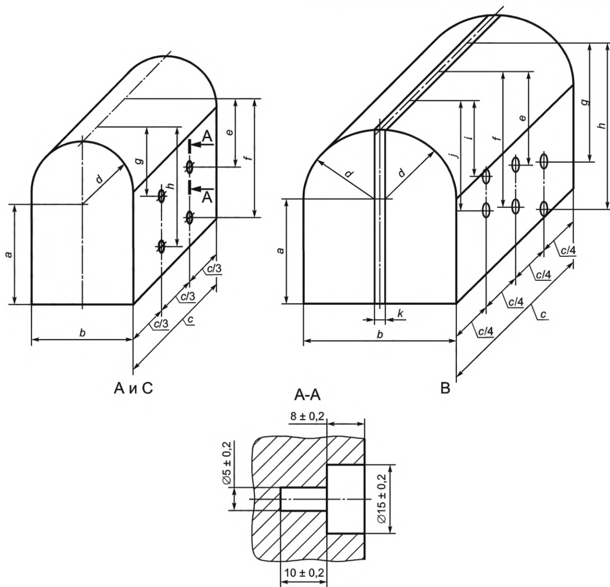
Размеры отверстия (сечение A-A)
