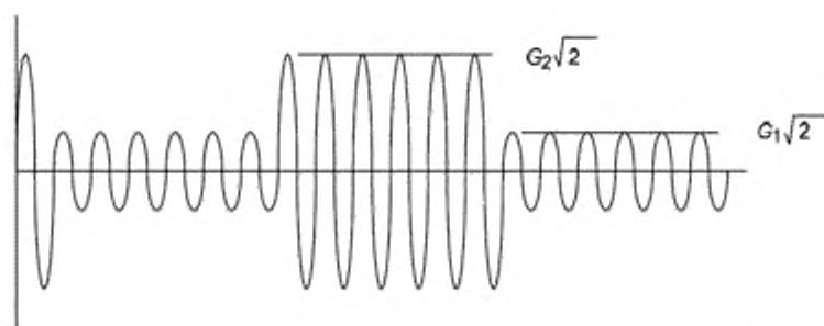
Рисунок 12 — Испытательная осциллограмма
