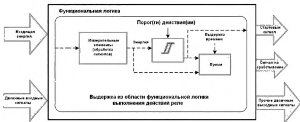
Рисунок 1 — Функциональный блок диаграмм выполнения защиты
