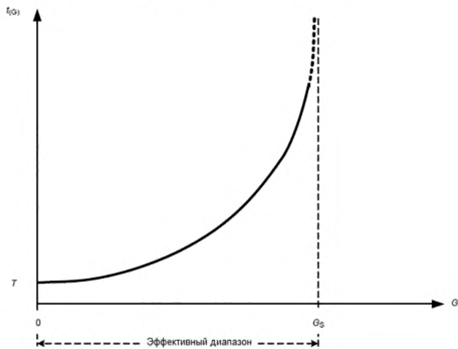
Рисунок 5 — Зависимость характеристики времени для защиты от недостаточного напряжения
