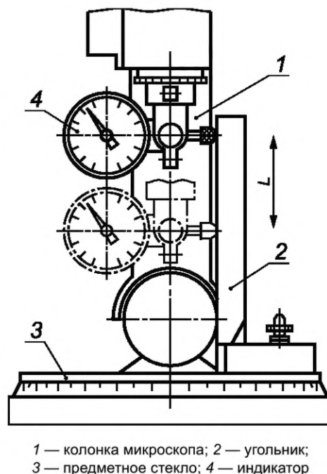
Рисунок 3 — Проверка прямолинейности движения тубуса микроскопа при перемещении механизмом точной фокусировки
