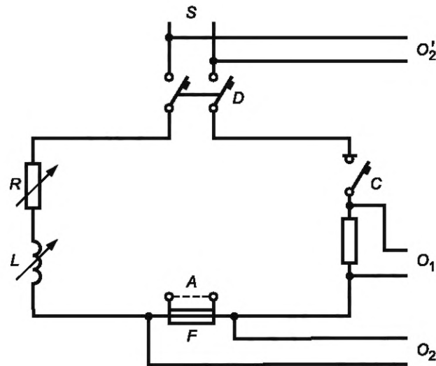
A — съемная перемычка применяемая при калибровке испытательной цепи; C — замыкающий выключатель; D — автоматический выключатель или другой защитный аппарат для защиты от пробоя; F — испытуемый плавкий предохранитель; L — настраиваемая катушка индуктивности; O_1 — измеритель для записи тока; O_2 — измеритель для записи напряжения при испытании; O'_2 — измеритель для записи напряжения при настройке; R — настраиваемое активное сопротивление; S — источник питания
