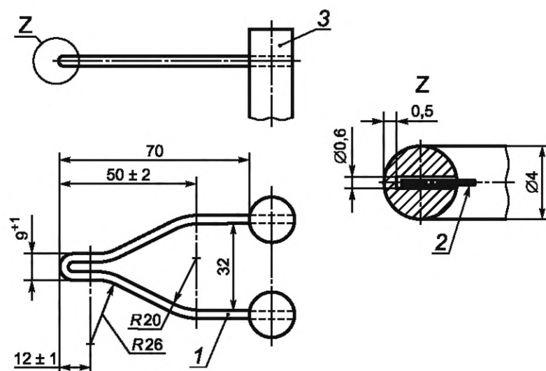
1 — раскаляемая проволока, припаянная к штифту 3; 2 — термопара; 3 — штифт
