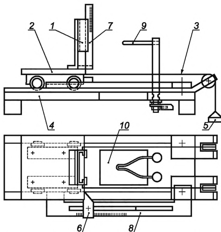
1 — опора для образца; 2 — тележка; 3 — натяжной канат; 4 — фундаментная плита; 5 — груз; 6 — регулируемый упор; 7 — линейка для измерения пламени; 8 — линейка для измерения проникновения; 9 — петля из раскаляемой проволоки (см. рисунок 8); 10 — отверстие в основании
