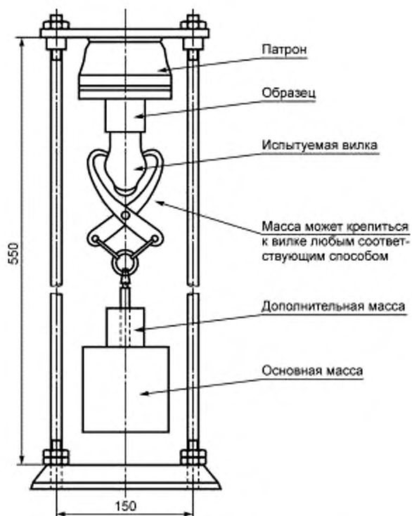
Рисунок 102 — Пример прибора для испытания усилия извлечения
