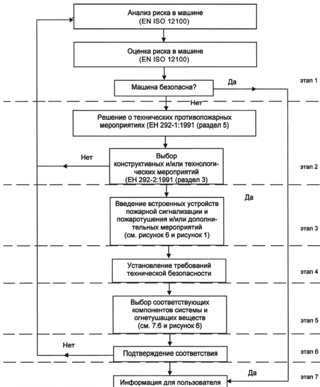
Рисунок 4 — Итеративный процесс выбора технических противопожарных мероприятий
