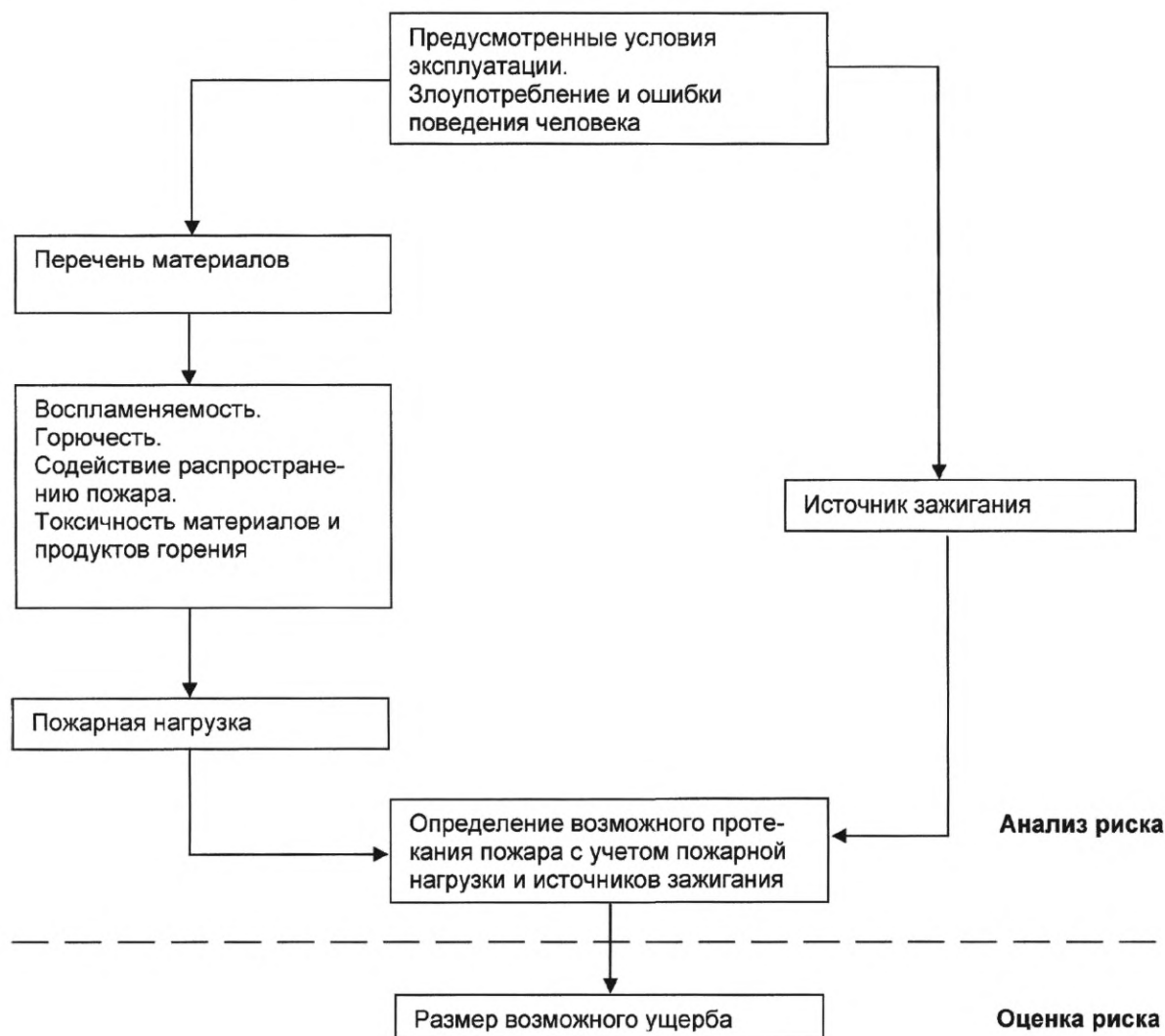
Рисунок 3 — Анализ и оценка риска
