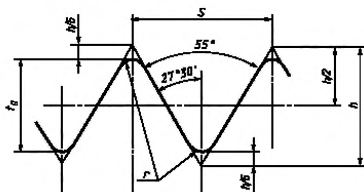
Трубная резьба ИСО
