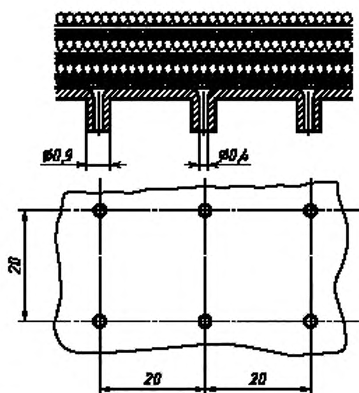
Рисунок 17 — Установка для проверки защиты от капель воды
