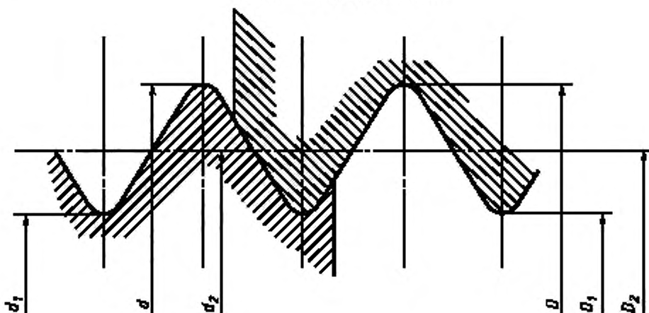
Предельный профиль винта
