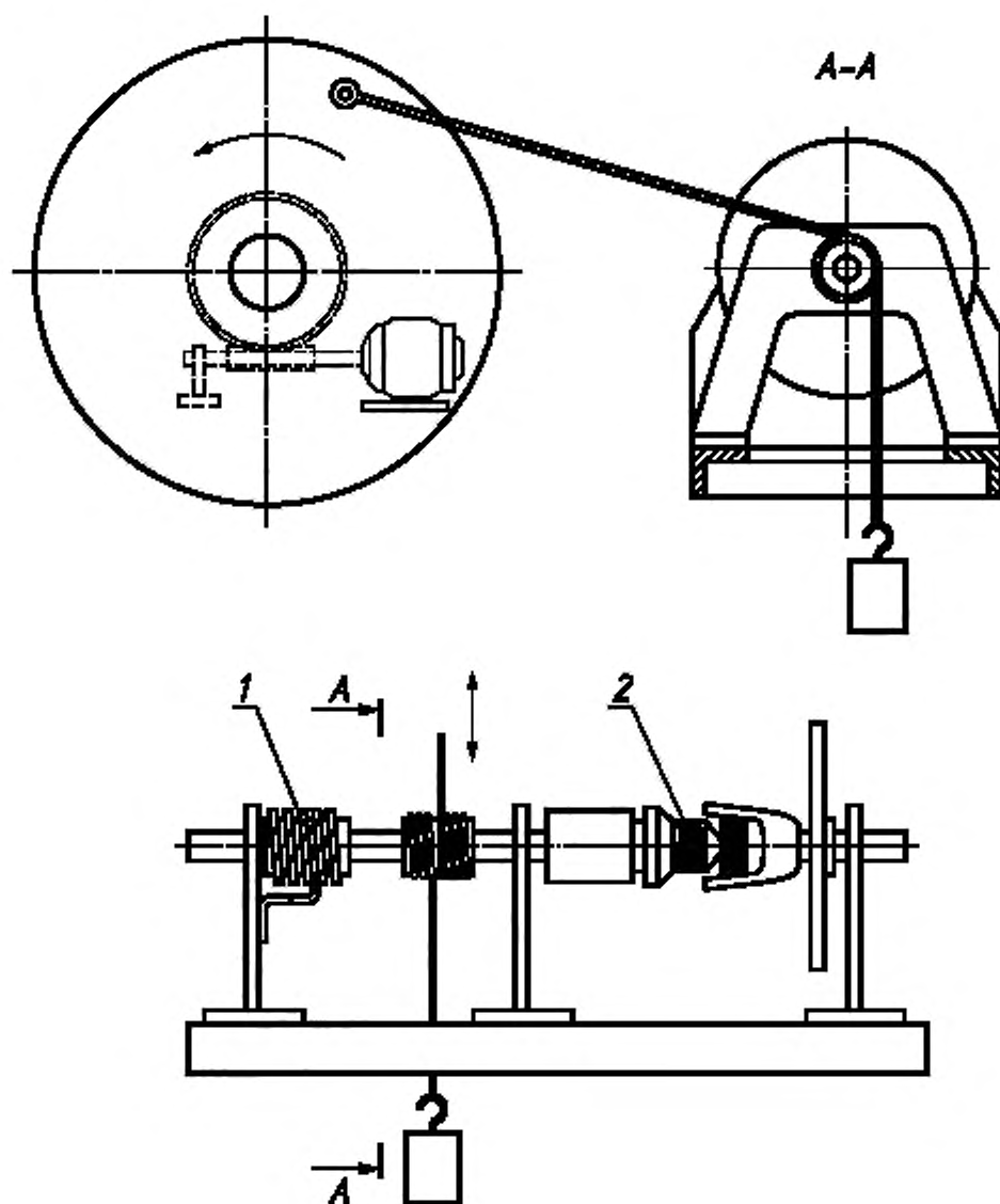
Рисунок 4 — Установка для проверки нормальной работоспособности
