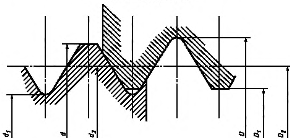
Предельный профиль винта
