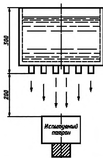
Рисунок 17 — Установка для проверки защиты от капель воды
