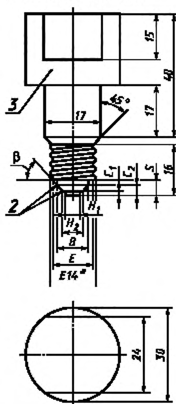
Испытательный цокль В
