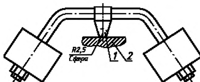
Рисунок 9 — Установка для испытания на сжатие
