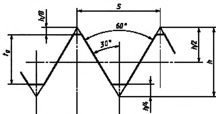
Основной и предельный профили для гайки и винта Метрическая резьба ИСО
