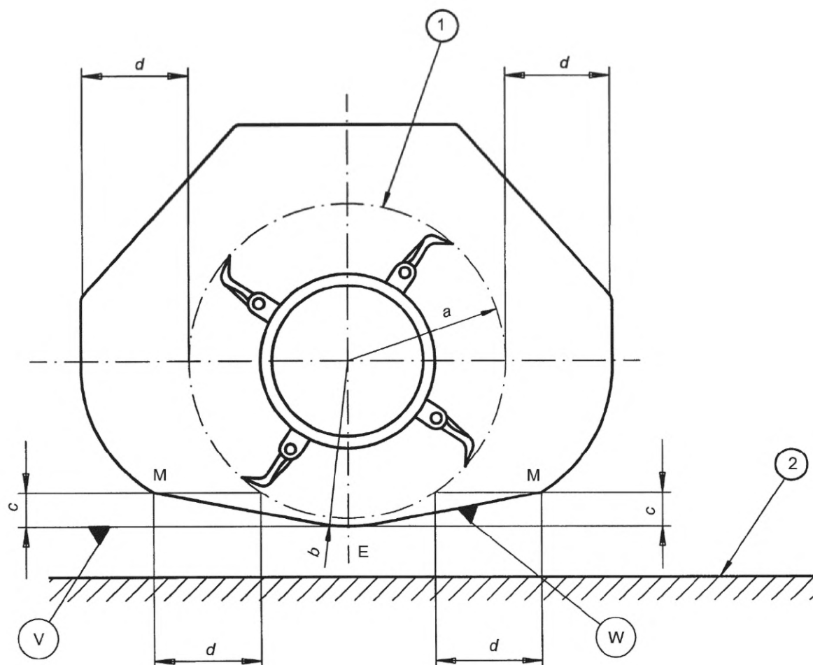
1 — траектория движения рабочего органа; 2 — почва; a — радиус траектории движения рабочего органа; b — радиус траектории движения рабочего органа не менее 3 мм; c — расстояние между точкой M и линией V (не более 120 мм); d — горизонтальное безопасное расстояние не менее 150 мм от траектории движения рабочего органа; E — точка пересечения окружности радиусом b с вертикальной плоскостью, проходящей через ось вращения; V — горизонтальная линия, проходящая через точку E ; W — линия, проходящая через точку M и касательная к окружности радиусом b
