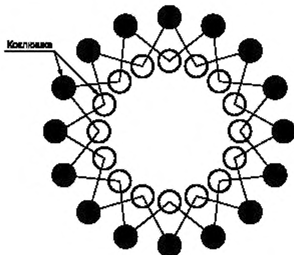
Рисунок В.1 — Текстильная оплетка
