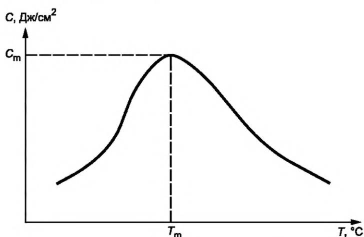
Рисунок 1 — Зависимость когезии от температуры
