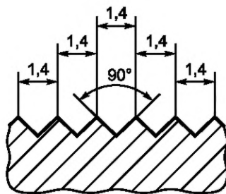
Рисунок 5 — Типичная форма зазубрин куба и подставки
