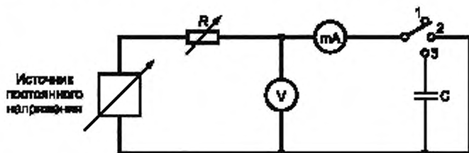
Рисунок 1 — Испытательная установка для выдержки при постоянном напряжении
