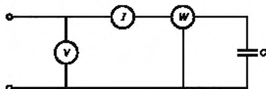
Рисунок 4 — Испытательная схема для измерения емкости и коэффициента мощности
