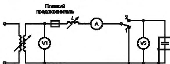
Рисунок 2 — Испытательная установка для разрушающего испытания переменным напряжением
