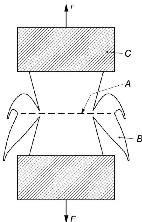
Рисунок В.4 — Закрепление трапецевидной испытуемой пробы, представленной на рисунке В.1
