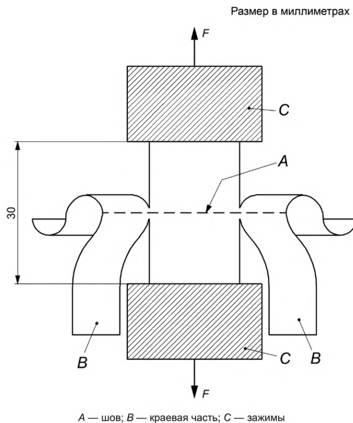
Рисунок В.3 — Закрепление прямоугольной испытуемой пробы, представленной на рисунке В.1
