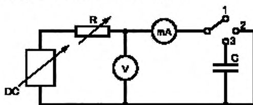
DC — источник постоянного напряжения; R — переменный резистор; V — вольтметр, mA — амперметр; 1, 2, 3 — положения переключателя; C — испытуемый конденсатор
