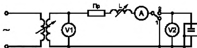
Пр — тугоплавкий предохранитель; L — регулируемая катушка индуктивности; V1 и V2 — вольтметры, A — амперметр
