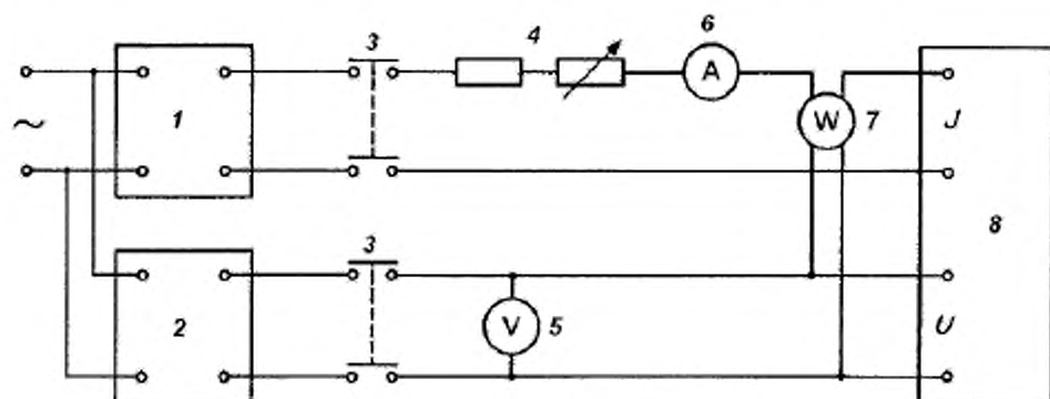
1 — источник меняемого напряжения, 2 — источник меняемого напряжения со сдвигом фаз; 3 — выключающее устройство; 4 — последовательный резистор; 5 — вольтметр; 6 — амперметр; 7 — ваттметр или счетчик коэффициента мощности; 8 — испытуемое реле
