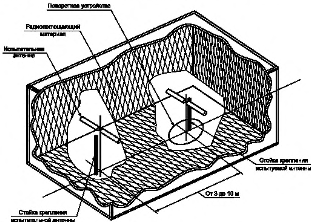
Рисунок А.1 — Пример типовой безэховой камеры
