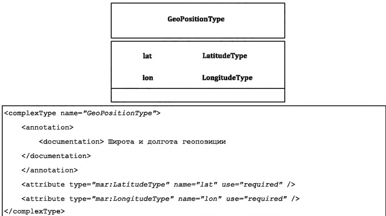
Рисунок 32 — Тип GeoPosition
