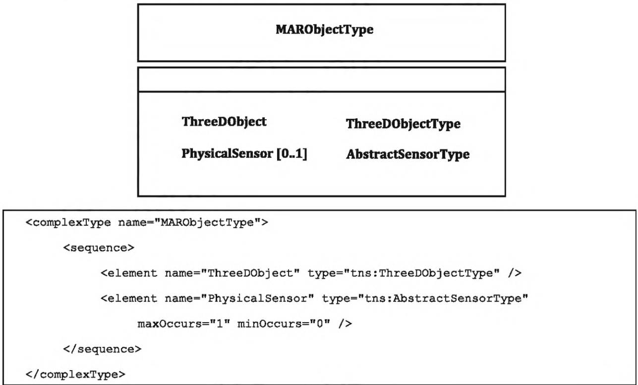
Рисунок 37 — Тип MARObject
