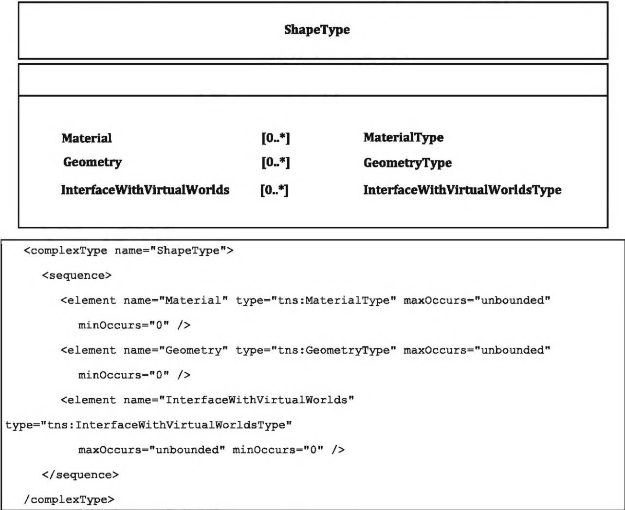
Рисунок 39 — Тип формы
