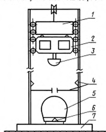
1 — устройство для подъема и сбрасывания каретки с ударником; 2 — каретка; 3 — ударник; 4 — устройство для измерения скорости падения каретки с ударником; 5 — макет головы; 6 — датчик; 7 — основание стенда
