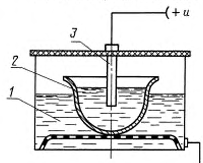
1 — электролит; 2 — корпус каски; 3 — подвижной электрод
