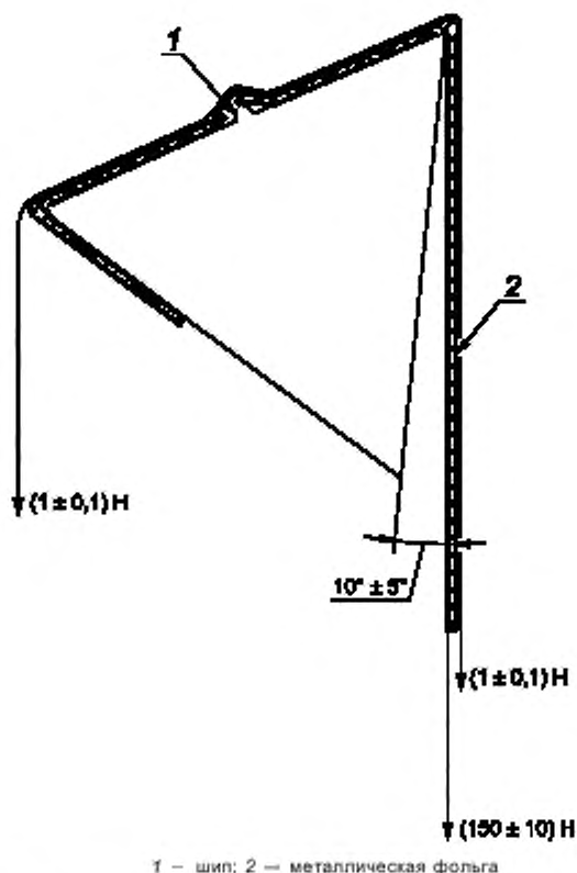
Рисунок 16 — Конечное положение оправки
