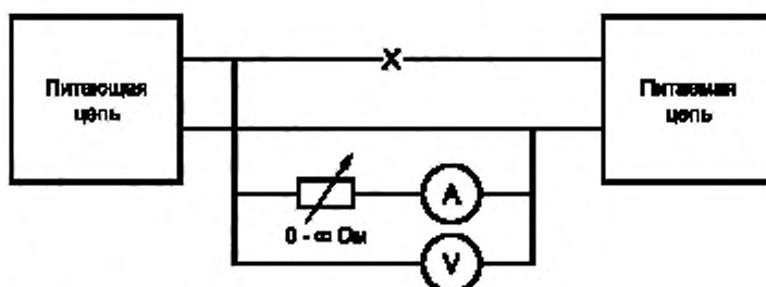
Рисунок 1 — Схема испытательной цепи для условий неисправности
