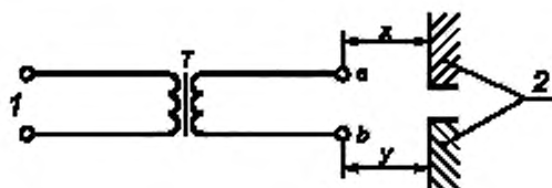
1 — сеть питания, 2 — электрически разделенные доступные проводящие части
