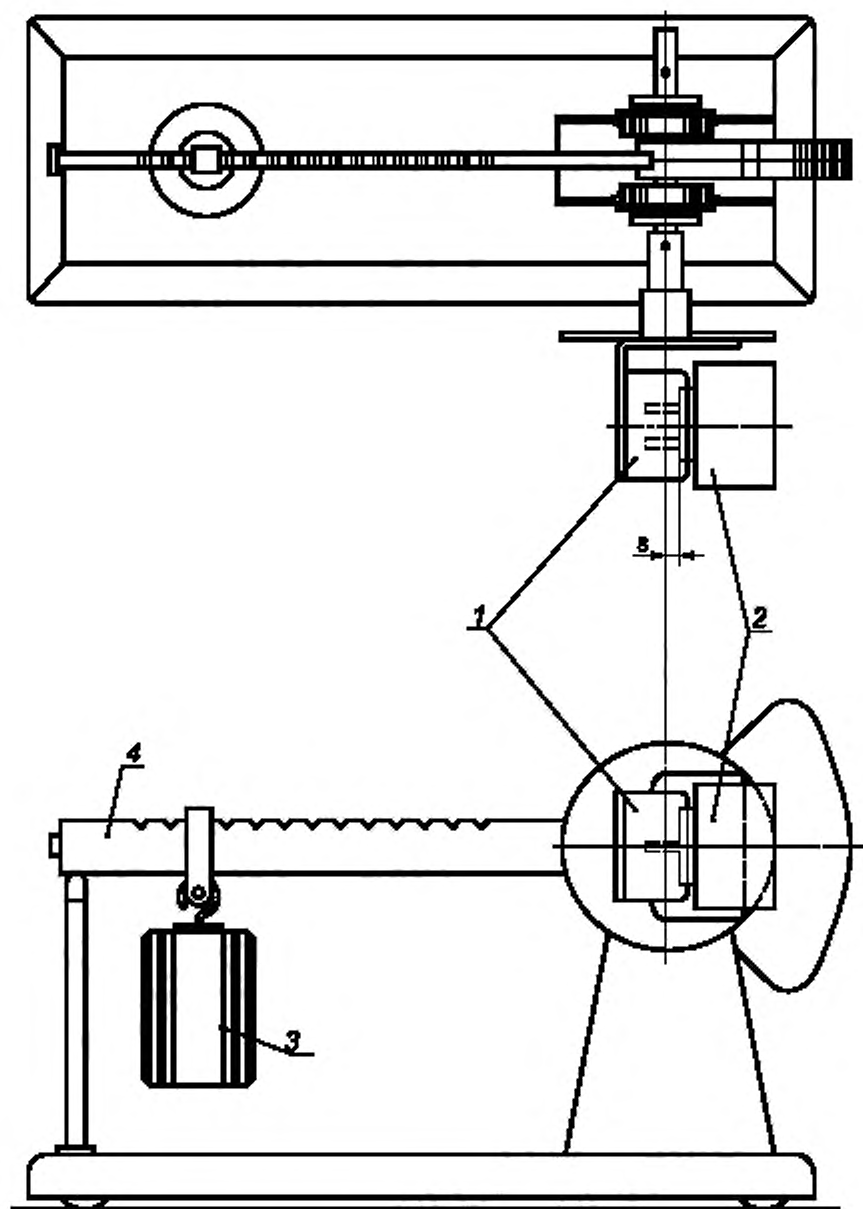
1 — розетка; 2 — образец; 3 — груз; 4 — балансирующий рычаг
