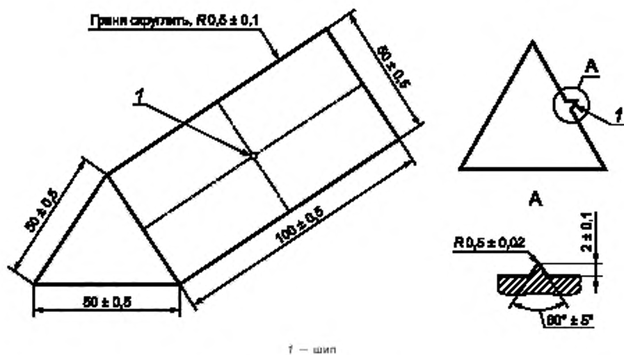
Рисунок 14 — Оправка
