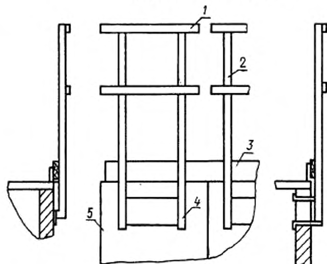
Защитное наружное опорное ограждение (Ограждение Зщ Нж Оп ГОСТ 12.4.059—89)
