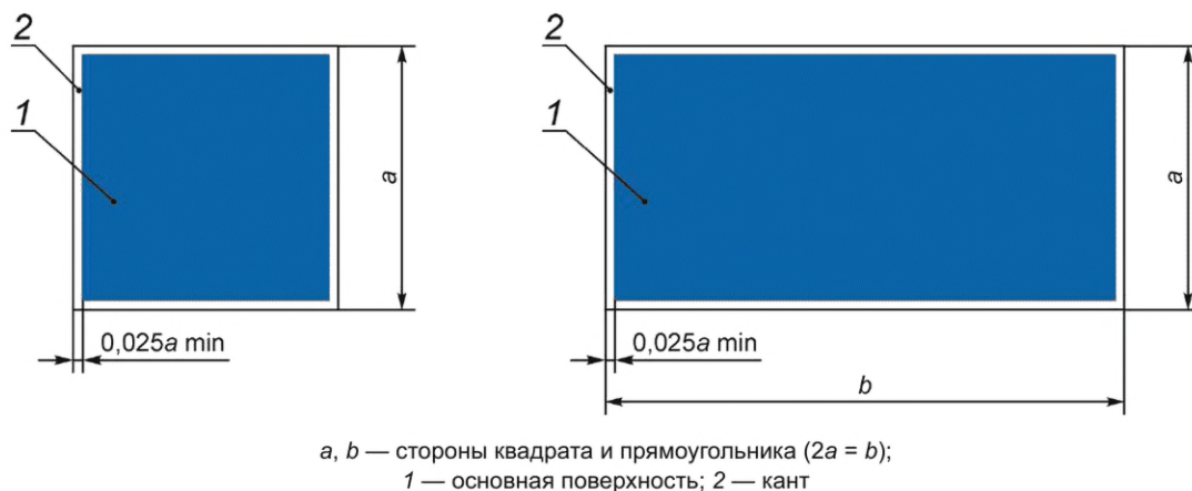
Рисунок 6 — Основа цветографического изображения и соотношение размеров указательных знаков безопасности
