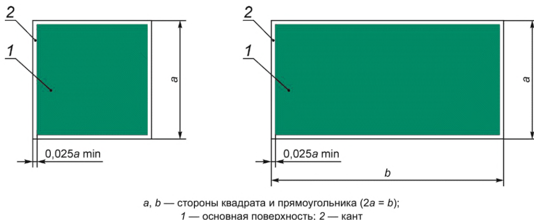
Рисунок 5 — Основа цветографического изображения и соотношение размеров эвакуационных знаков безопасности и знаков безопасности медицинского и санитарного назначения
